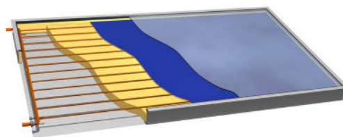
Genomskäring
